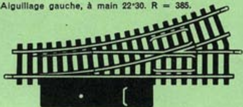
Réf. 85. Aiguillage gauche, à main 22°30'. R = 385.
