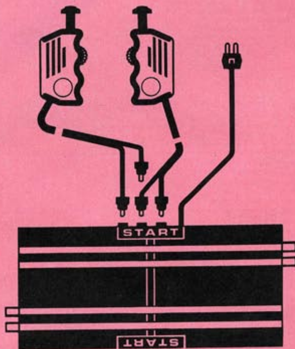
Réf. 310 A. Route d'alimentation. Longueur 260 mm. Composé de : 1 route; 2 poignées avec fils (amovibles).
